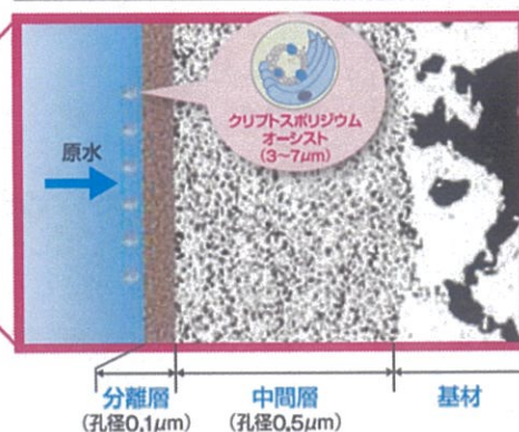
分離層と中間層のセラミック膜二重構造
