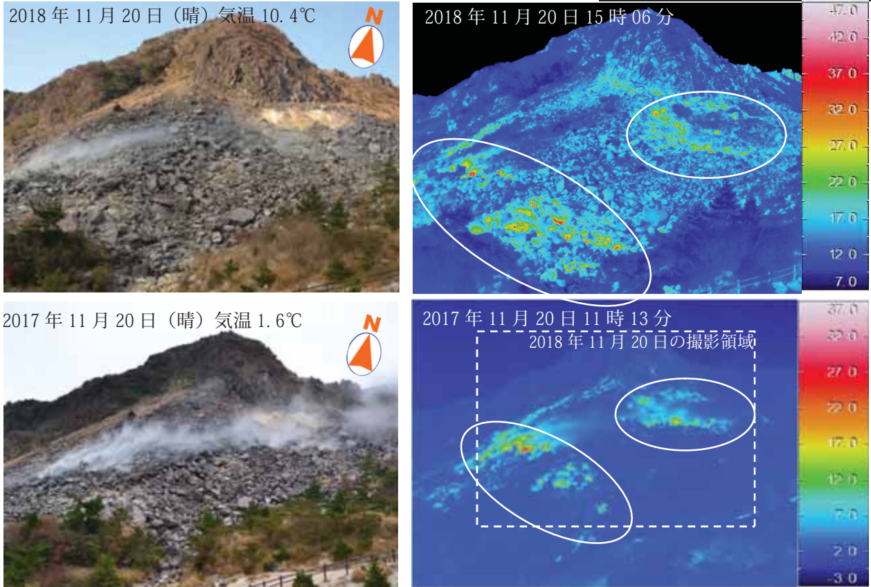
図5 鶴見岳・伽藍岳 伽藍岳噴気地帯の赤外熱映像装置による地表面温度分布 (図中の白丸は伽藍岳噴気地帯の熱異常域を示す)
