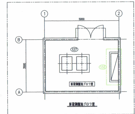
宇佐市不燃物処理場 浸出水処理施設更新工事 機器配置図（水槽上屋平面図） （更新工事後）
